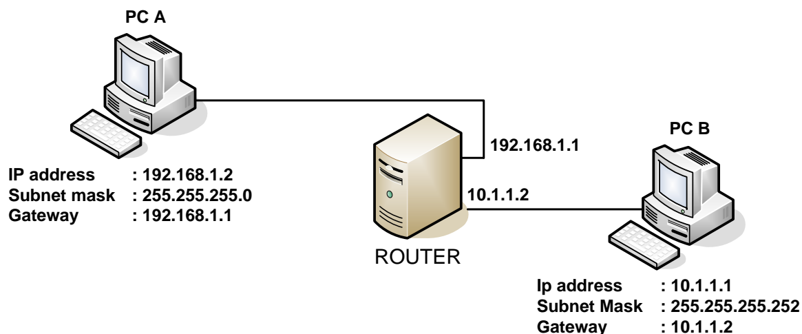
Gambar 2.4 Konfigurasi Jaringan
