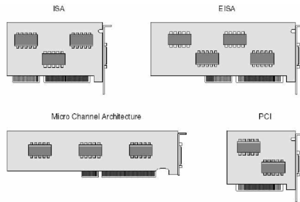
Gambar 1.1 Kartu Jaringan
